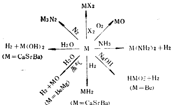
图13-2 碱土金属的一些化学反应
