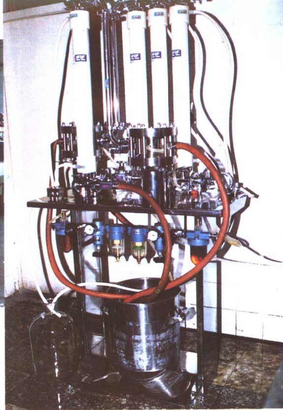
▲ 天津纺织工学院研制成功聚砜中空超滤装置 李跃平 摄
