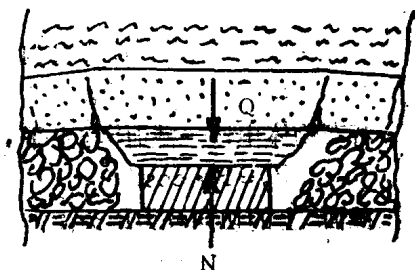
图1-2 煤柱受压状态
