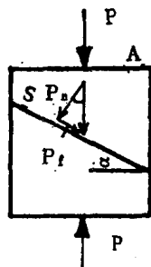
图1-3 应力分析图
