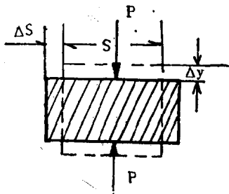
图1-5 压缩变形
