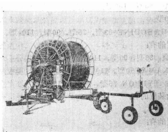
图11 “BERGNMGSMASCHINE 90/300” 绞盘式喷灌机（活塞驱动）
