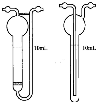
(a) 多孔玻璃吸收瓶 (b) 氧化瓶
