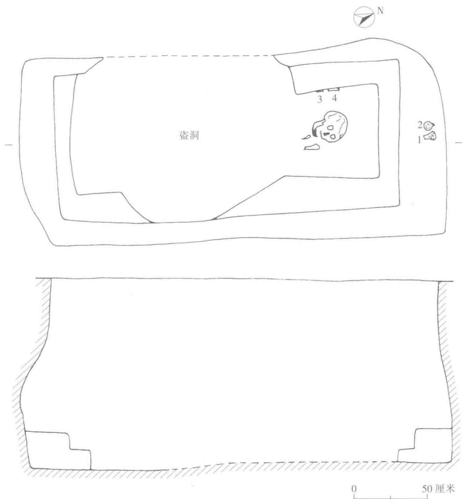
图 2-221A SM27 平、剖面图
