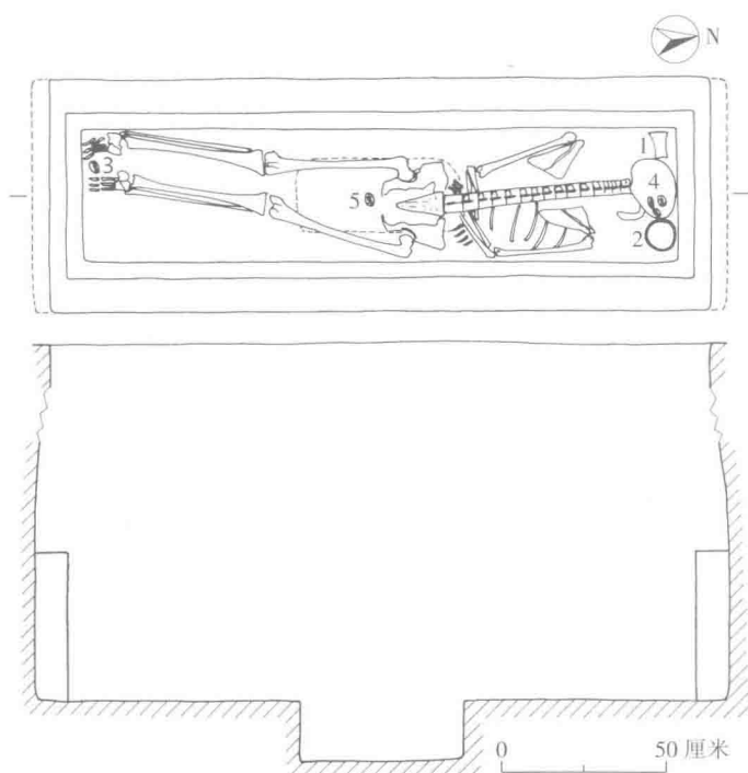
图 2-225A SM62 平、剖面图
