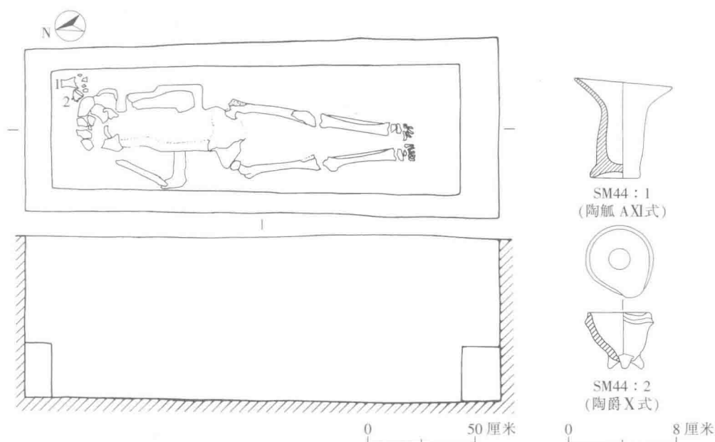
图 2-224 SM44 平、剖面图及出土遗物
