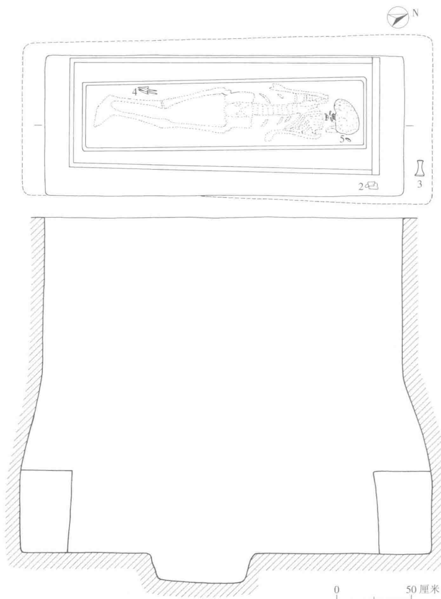
图2-223A SM29平、剖面图
