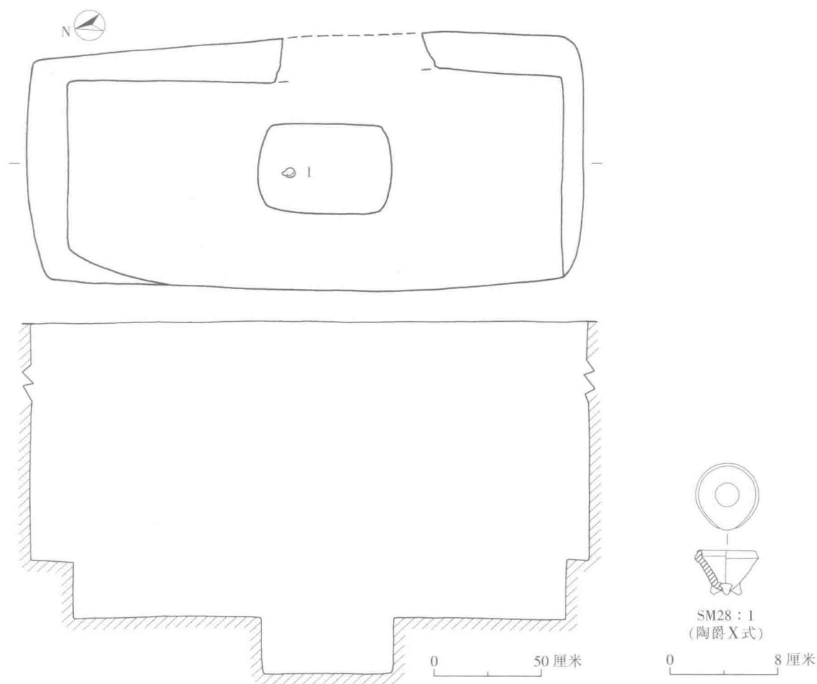
图 2-222 SM28 平、剖面图及出土遗物
