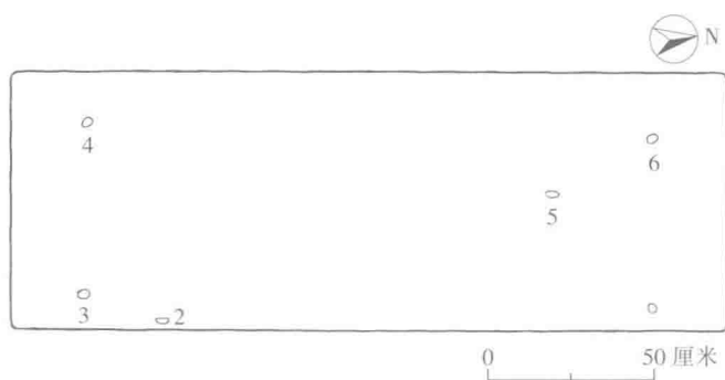
图 2-225B SM62 墓底桩孔图
