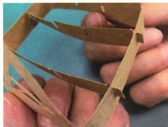
5 ⑧的两端分别插入③和④的底部的“U”型槽中。
