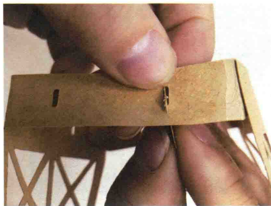
4 ⑦的两端分别插入③和④的底部的“U”型槽中。
