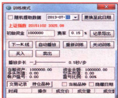
图 X-1 训练模式
