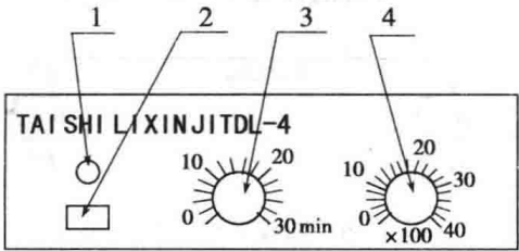
1. 电源指示灯 2. 电源开关 3. 定时旋钮 4. 转速旋钮
