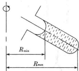
图 2-1 离心机的工作原理
