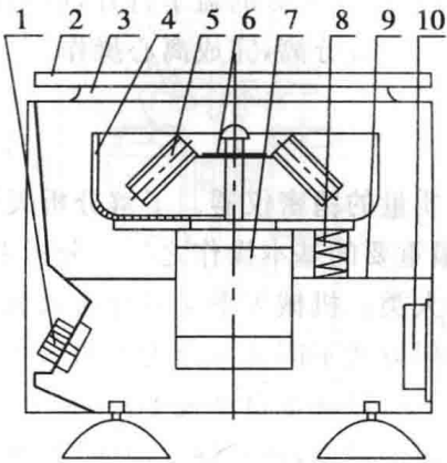
1. 控制面板 2. 盖板 3. 密封圈 4. 保护腔 5. 转子 6. 盖形螺母 7. 电机 8. 减震装置 9. 机架 10. 电机控制系统
