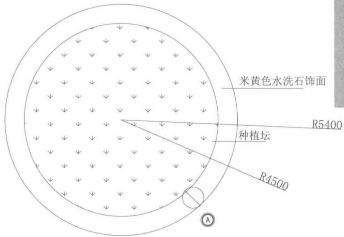
花坛平面图
