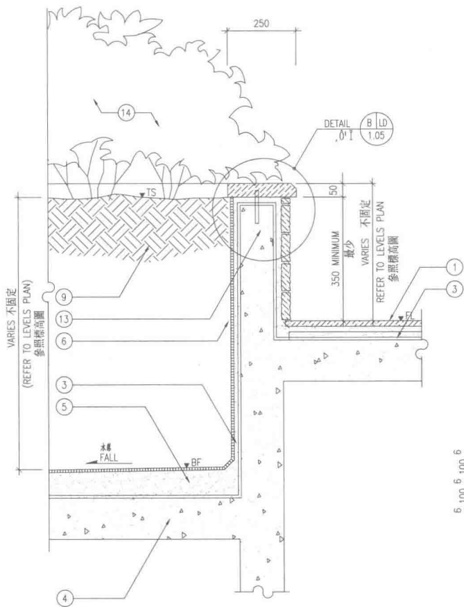
剖面图 1:10
