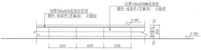
立面图 1:20
