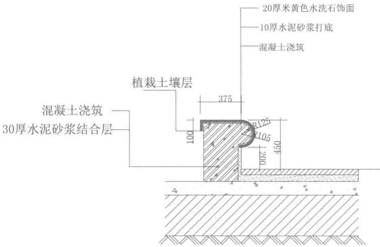
大样图
