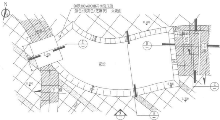
花坛平面图 1:50
