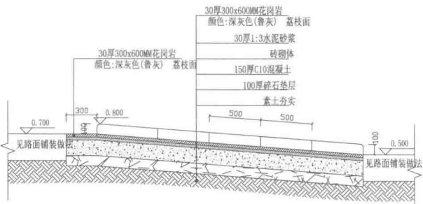
剖面图 1:20
