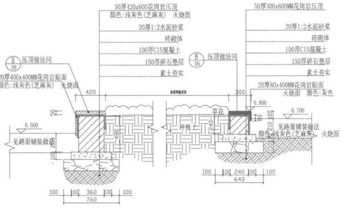
剖面图 1:20
