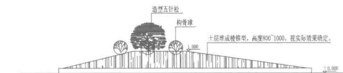
入口花坛侧立面图
