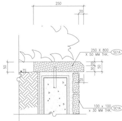
详图 1:5
