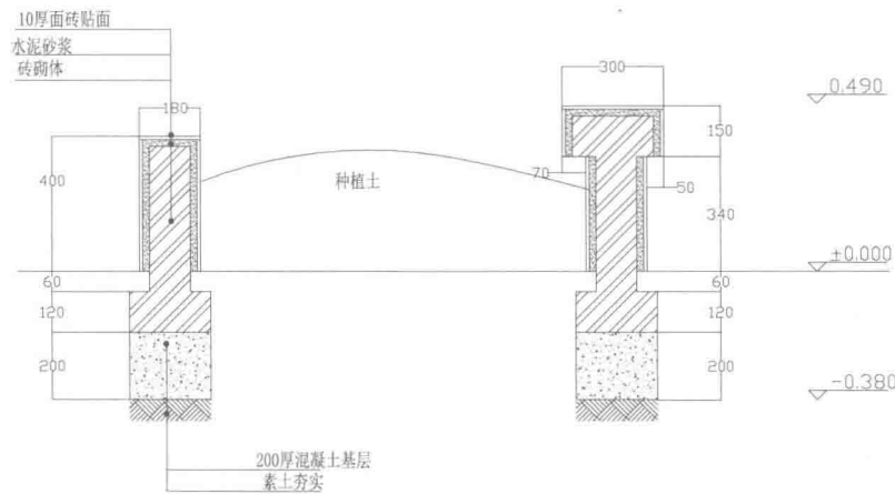
A-A剖面图
