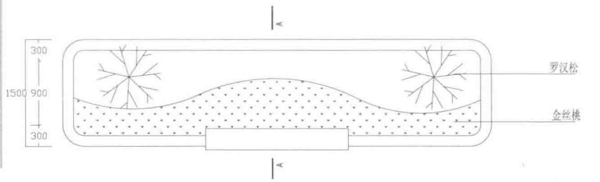
花坛平面图
