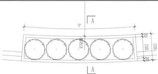
花坛平面图
