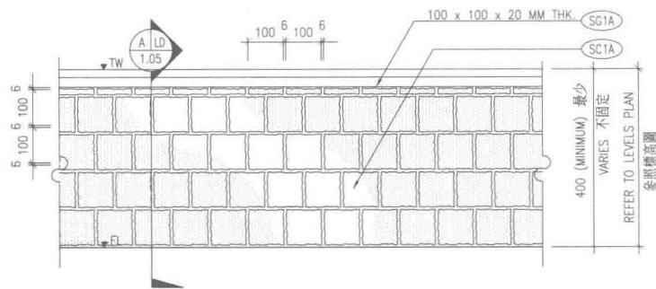
局部立面 1:10
