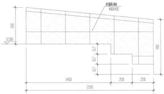
花坛侧立面图
