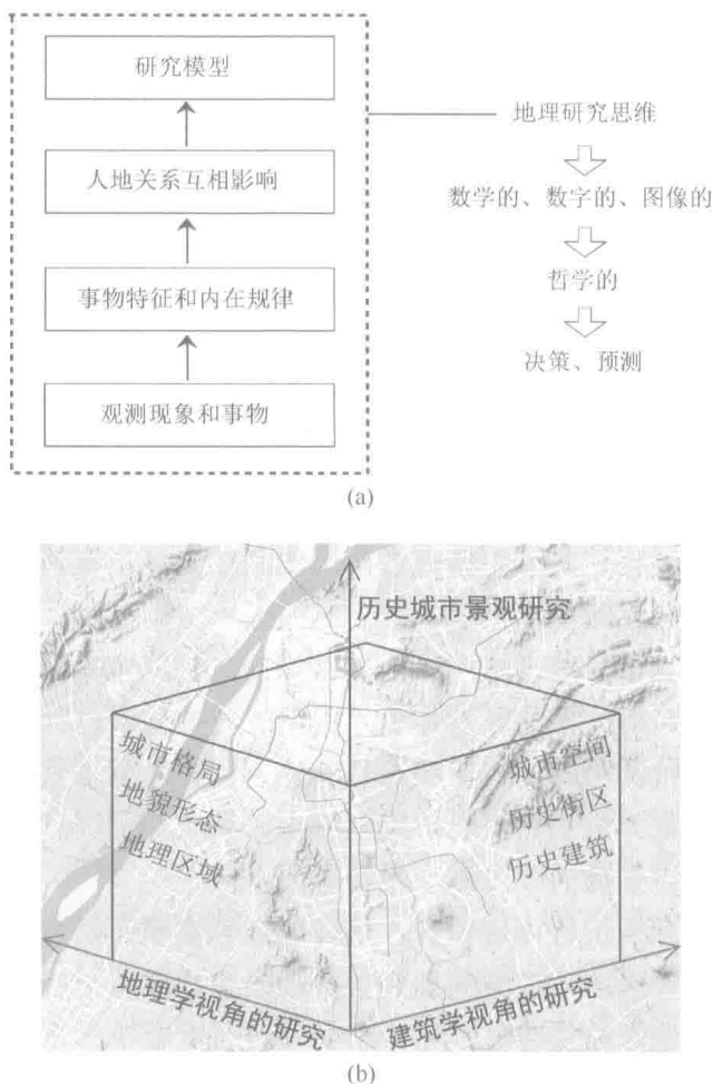
图 1.1 地理学与建筑学研究思路比较
