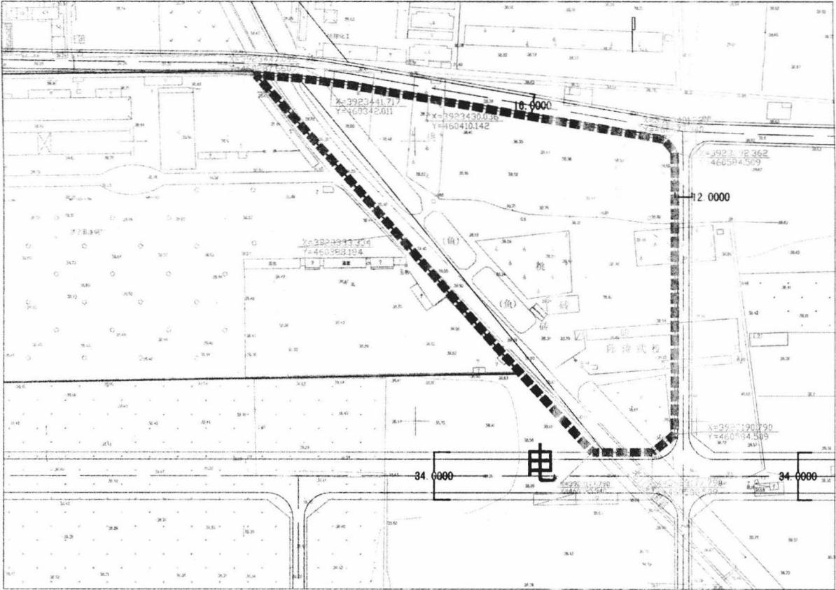
图 1-2 山东某新城中心区城市公共绿地：从现状图中可以分析出场地内部的一些情况，包括场地地形标高、现有建筑、鱼塘、桃树等
