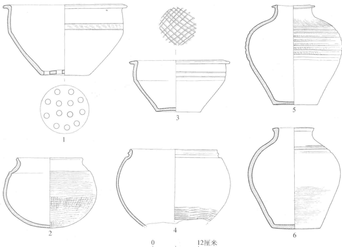
图三五四 SDM211、SDM213随葬陶器
