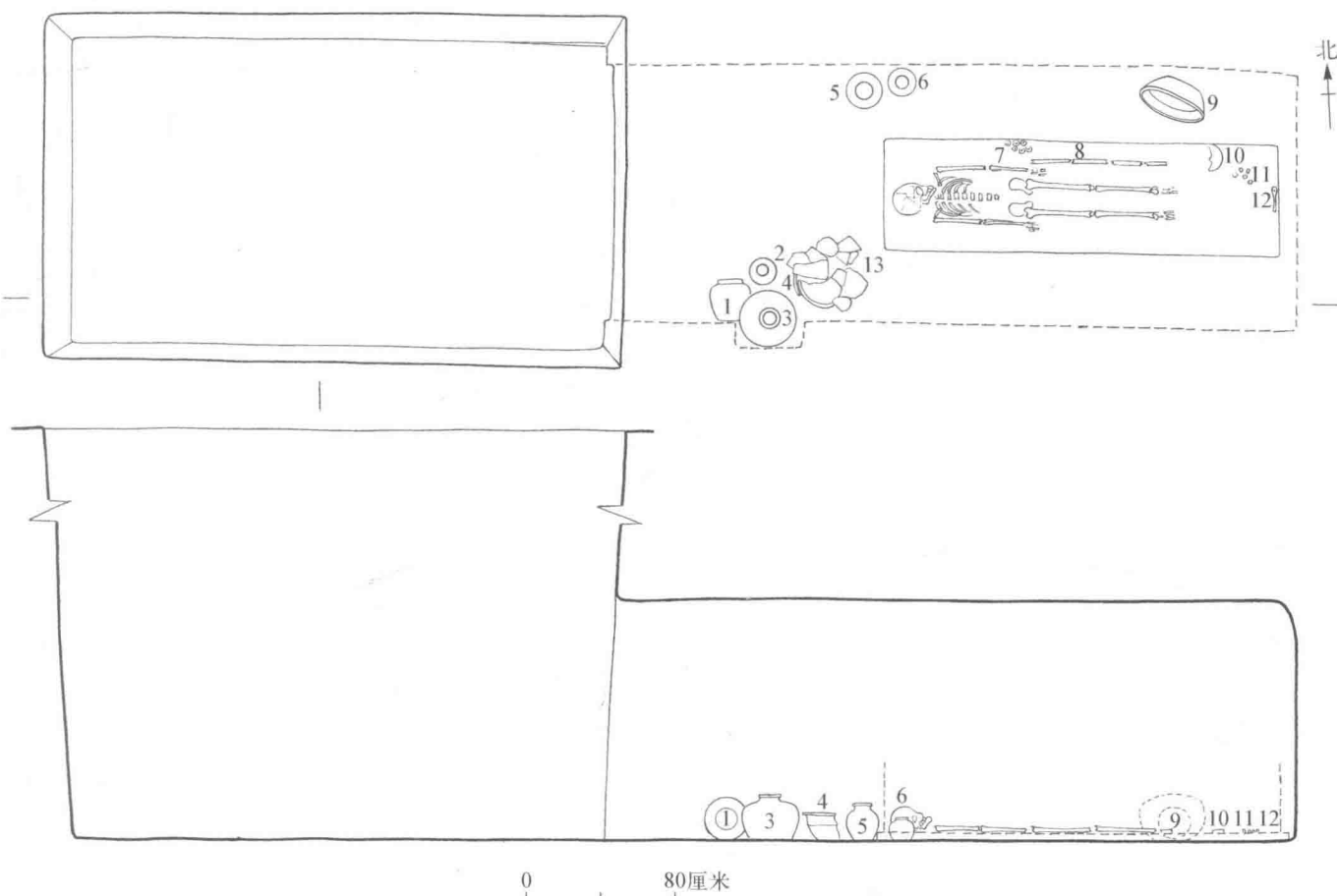
图三四八 SDM209墓葬平、剖图
