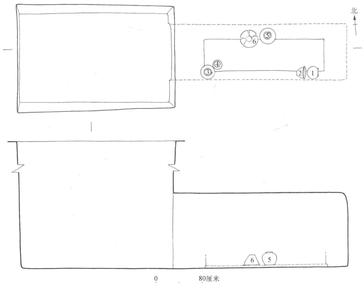
图三五二 SDM210墓葬平、剖图
