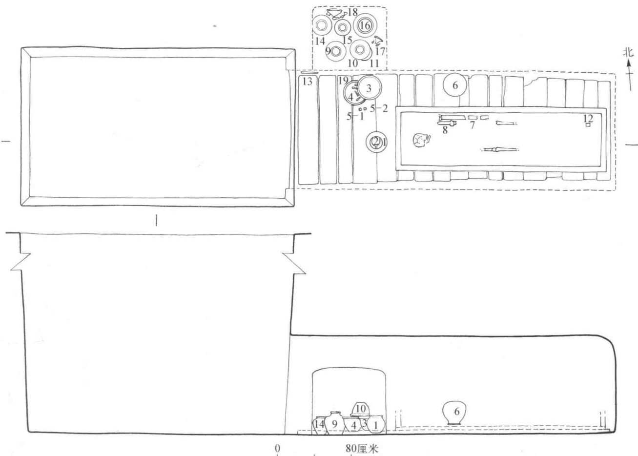
图三五五 SDM213墓葬平、剖图
