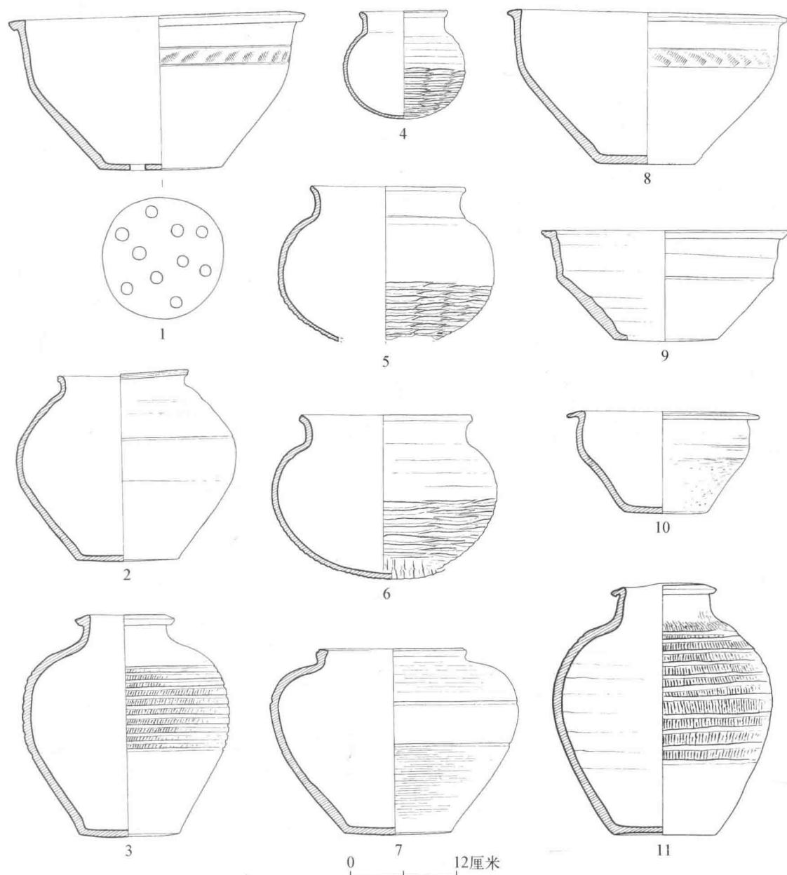
图三五〇 SDM209、SDM210随葬陶器
