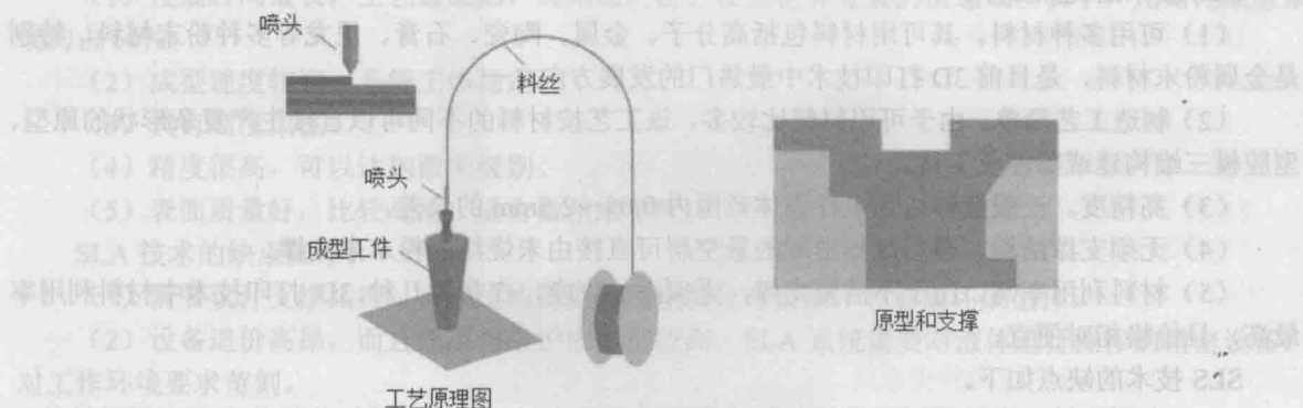
图 1-4 FDM 打印原理
