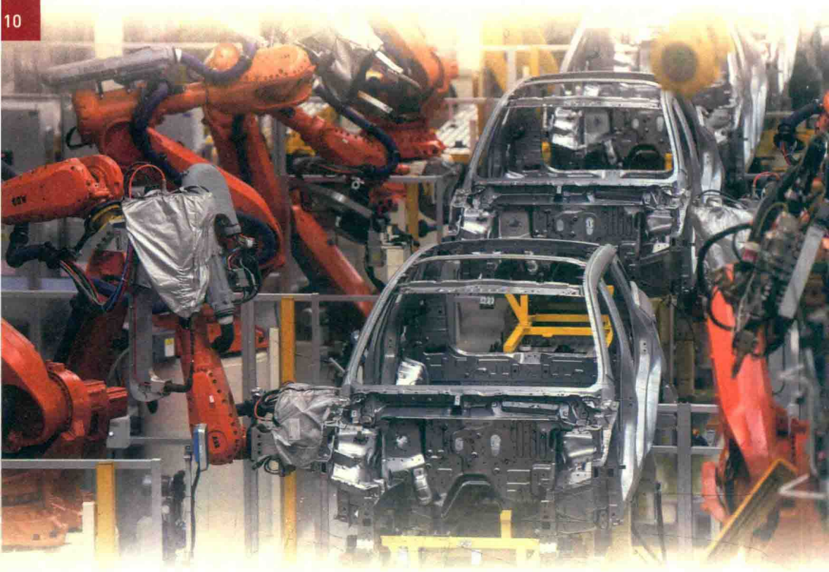
▲ 浙江省宁波市北仑区吉利汽车春晓制造基地的自动化焊接线（2018年10月25日摄）
