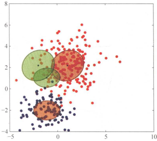
图 13.3 EM 算法用于 GMM 的示例
