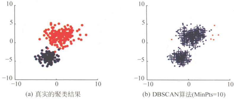
图 17.5 DBSCAN(MinPts=10)预测与真实结果对比
