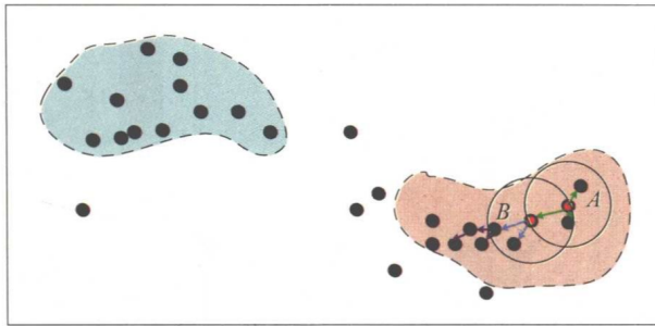
图 17.3 DBSCAN 算法聚类的过程
