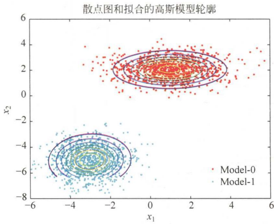
图 16.6 拟合高斯混合模型实例
