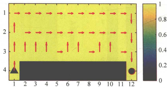
图 19.3 SARSA 算法得到的策略
