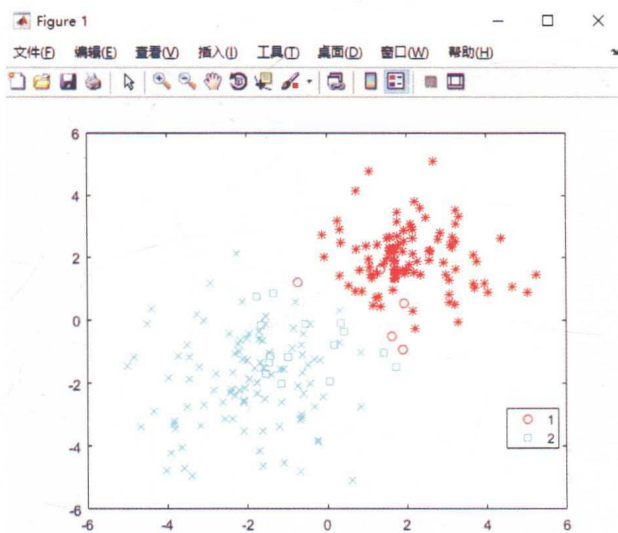
图 4.6 knnclassify 函数的 KNN 分类
