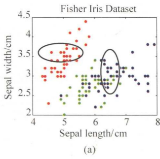
图 13.3 EM 算法用于 GMM 的示例
