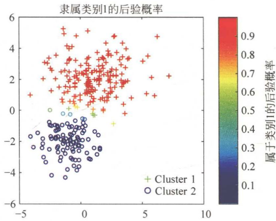
图 16.10 类别 1 的隶属度
