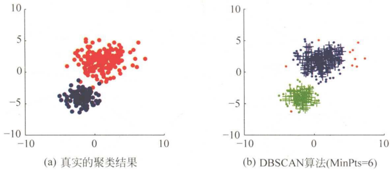
图 17.4 DBSCAN(MinPts=6)预测与真实结果对比
