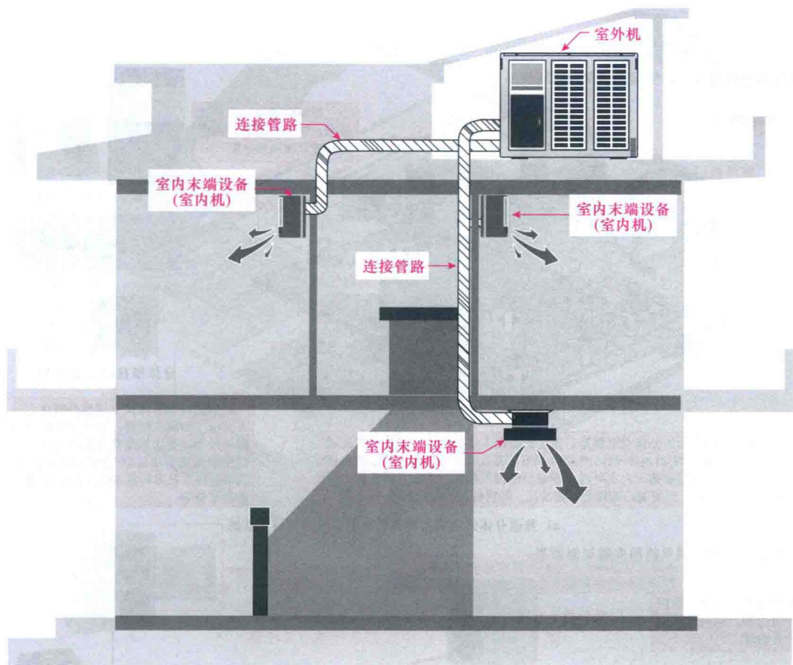
图 1-3 中央空调系统的应用
