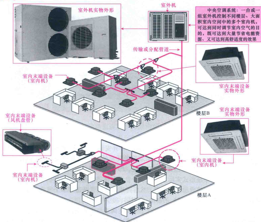
图 1-1 典型中央空调系统示意图
