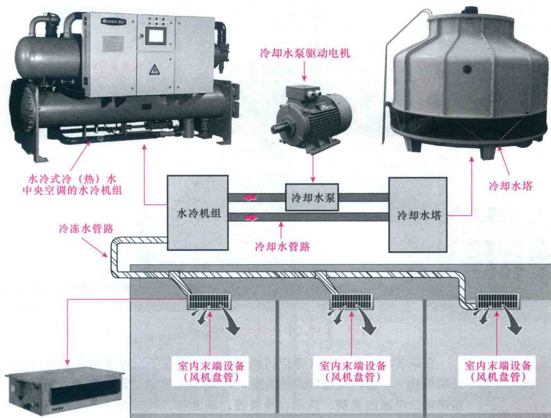
图 1-8 典型水冷式中央空调系统示意图
