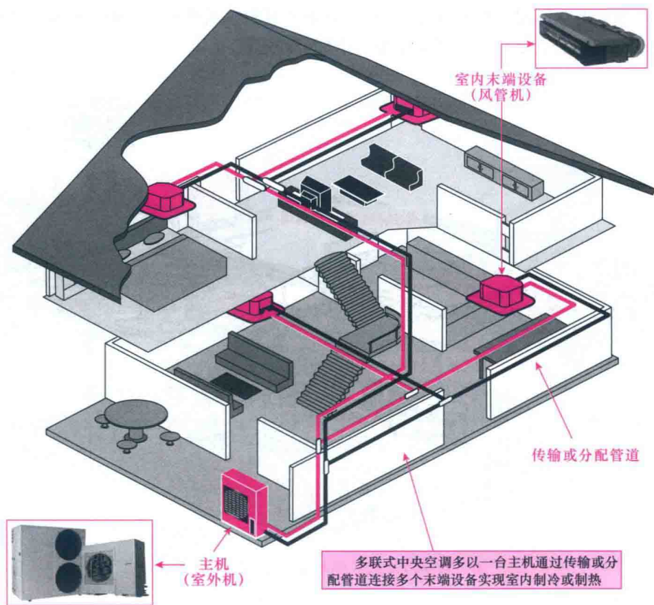
图 1-5 典型多联式中央空调系统示意图
