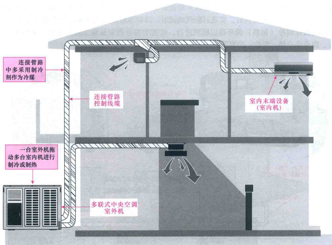
图 1-9 多联式中央空调的整体结构
