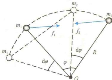
图 1-2 角动量守恒定理
