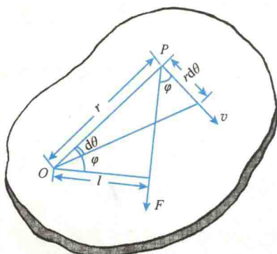
图 1-1 刚体的转动
