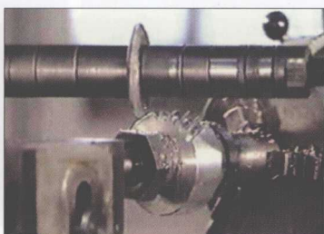
铣削斜齿轮
