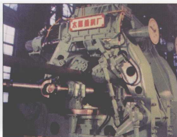
管材矫直生产
