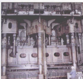
40MN汽车纵梁油压机
