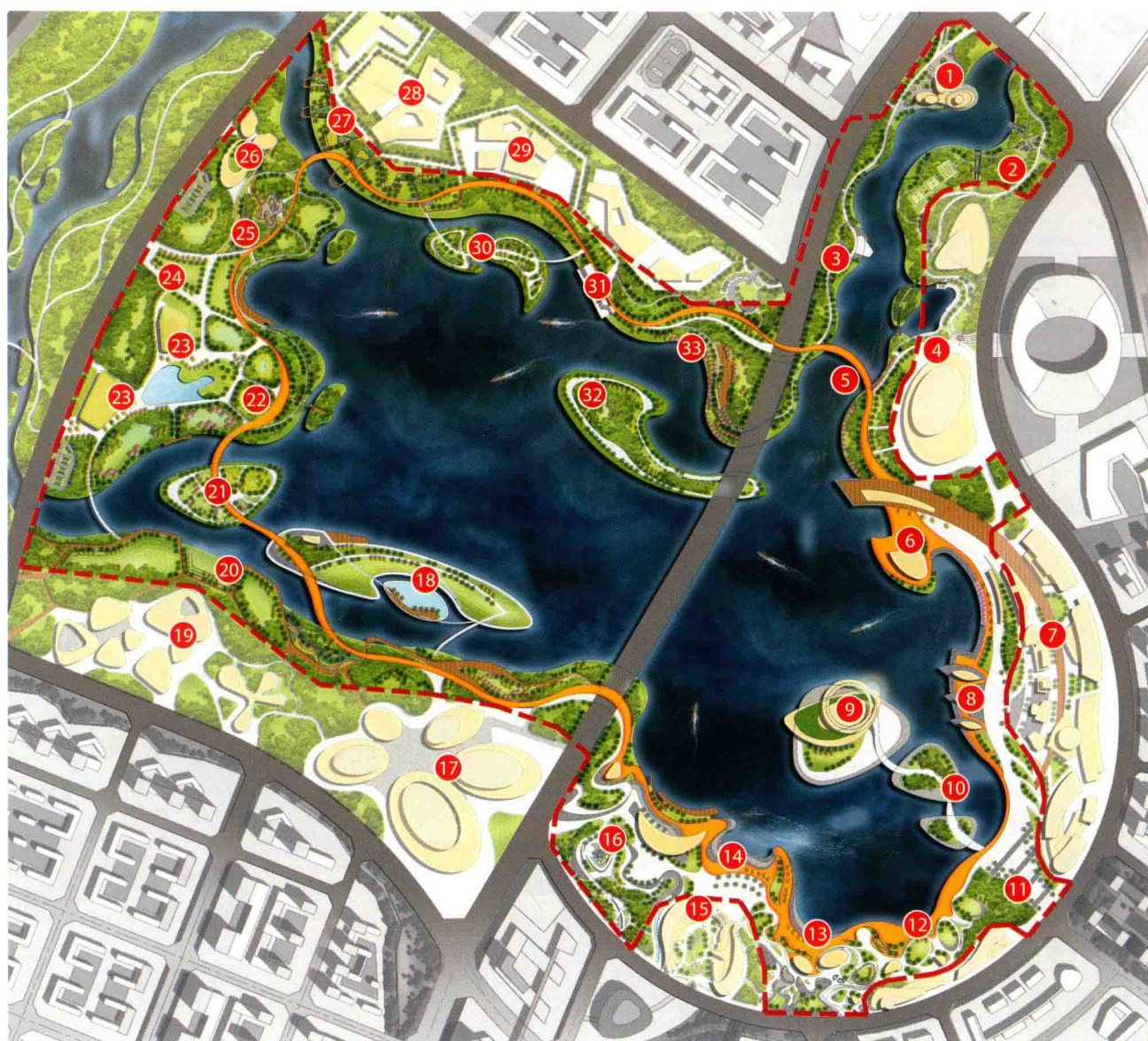
总平面图
