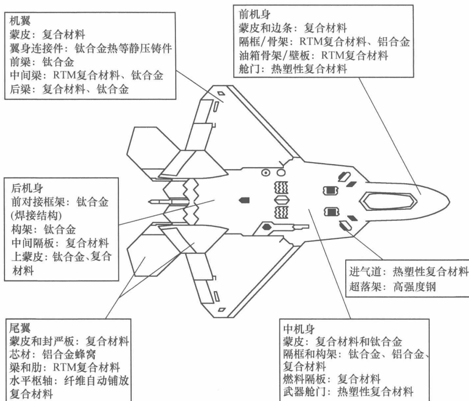
图 0-1 F22 战斗机上应用的工程材料
