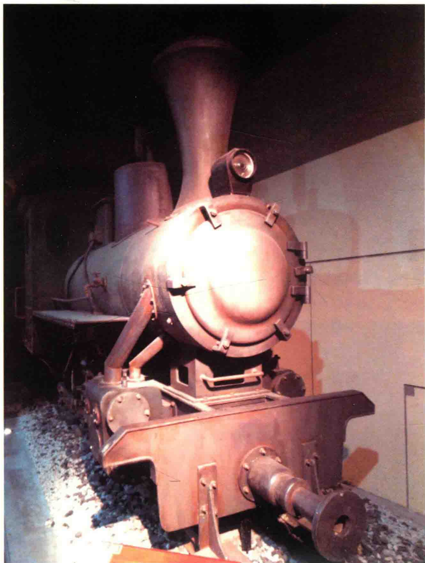
照片 7：天府煤矿自制蒸汽机车，作者摄于重庆中国三峡博物馆
