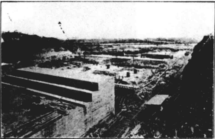
嘉敦閘西部之前灣及土臺
