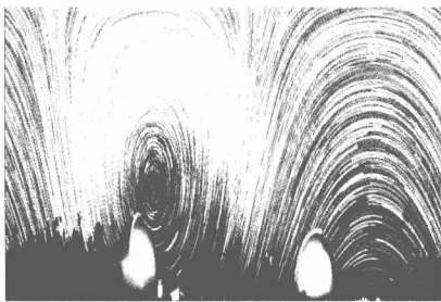
□ 时空弯曲
