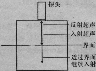
图 1-8 垂直入射时超声反射
