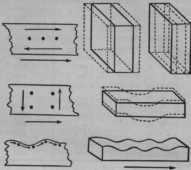
图 1-5 超声在固体中传播时的三种振态 上图: 纵波 中图: 横波 下图: 表面波
