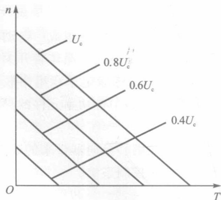
图 2.4 直流伺服电动机的机械特性
