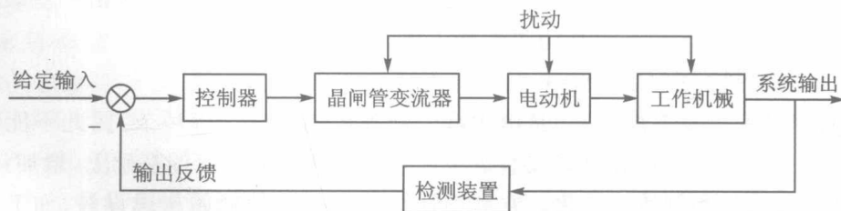
图 1.2 机电传动闭环控制系统
