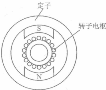
图 2.1 无槽电枢直流伺服电动机结构
