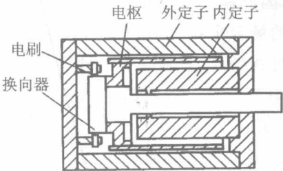
图 2.2 空心杯电枢直流伺服电动机结构
