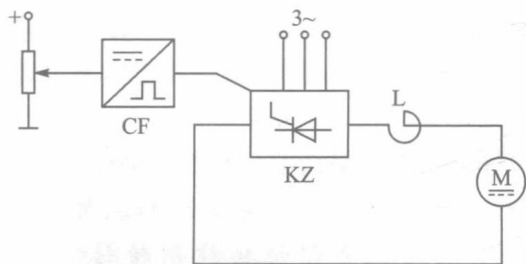
图 2.5 晶闸管直流调速驱动
