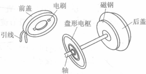
图 2.3 盘形电枢直流伺服电动机结构
