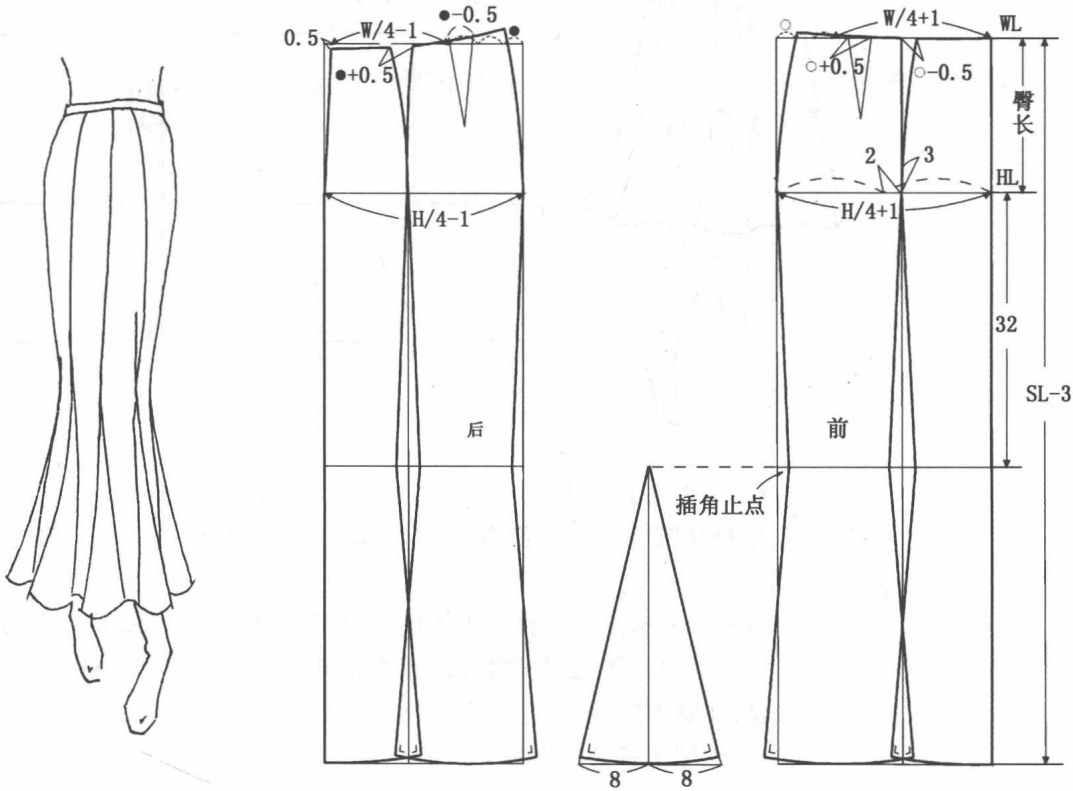
款式二：插角鱼尾波浪裙，其结构制图如图 1-3 所示。
