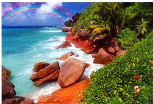
训练2-1 创建透明渐变
