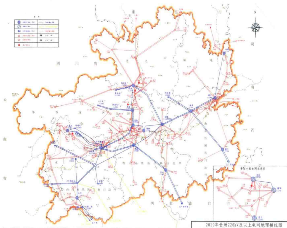
2010年贵州电网地理接线图
