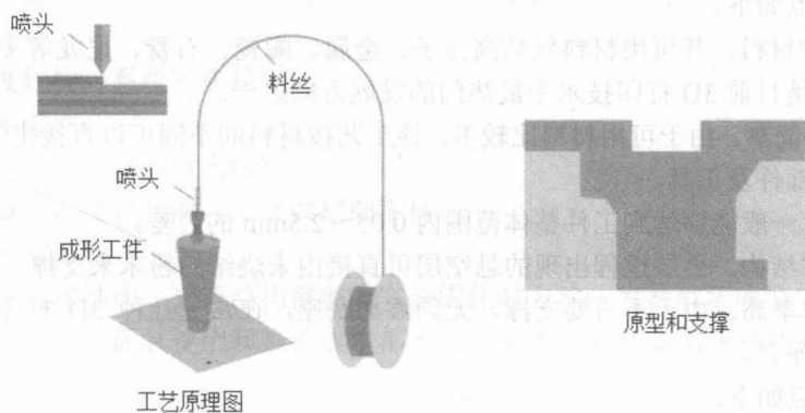
图 1-4 FDM 打印原理
