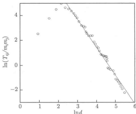
图 1.1 比利时铁路客运量中的引力定律 [3]
