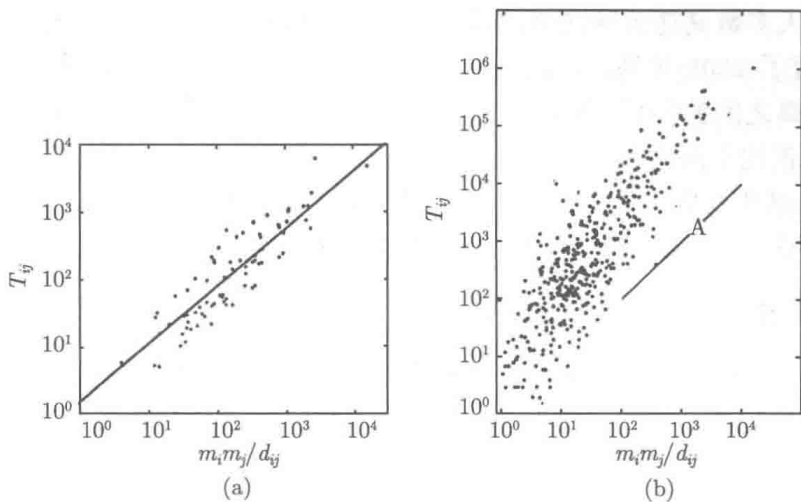
图 1.2 美国铁路网络中的引力定律 [7]
