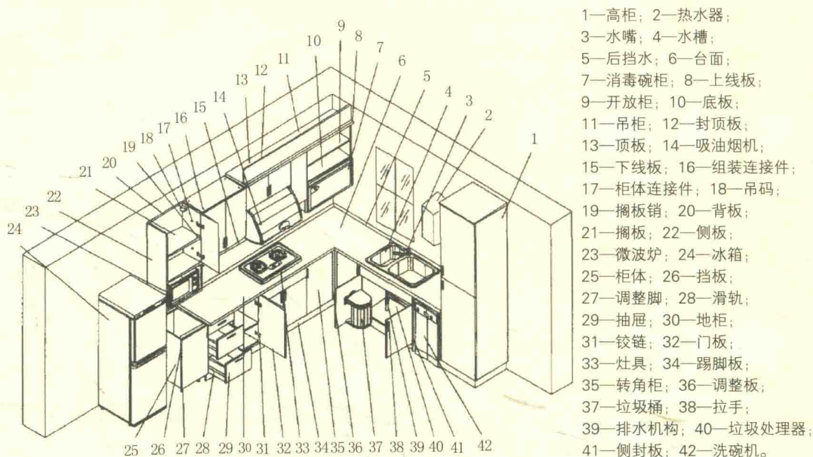
图1-1 家用厨房设备部件名称示意图
