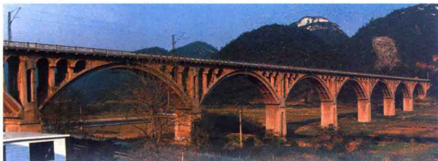
1979年8月建成的贵阳大土至湖潮铁路环线花溪大桥，为当时国内最长的双曲铁路拱桥
