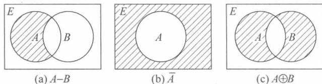
图 1.2 A-B, \bar{A}, A \oplus B 的文氏图
