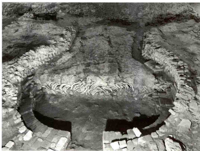
△ 珠山御窑厂葫芦窑遗址
