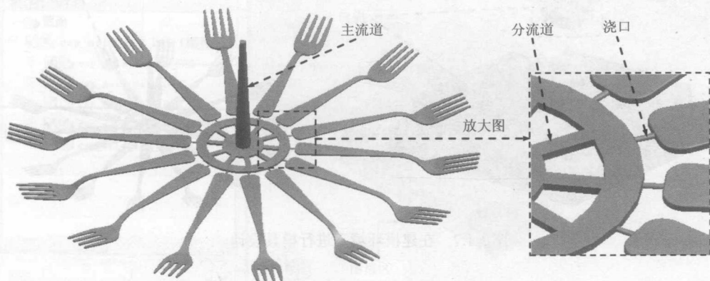
图 1.1.5 浇注系统
