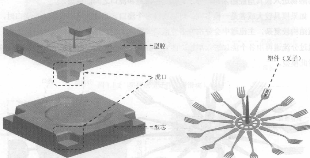
图 1.1.7 在建模环境下进行模具设计
