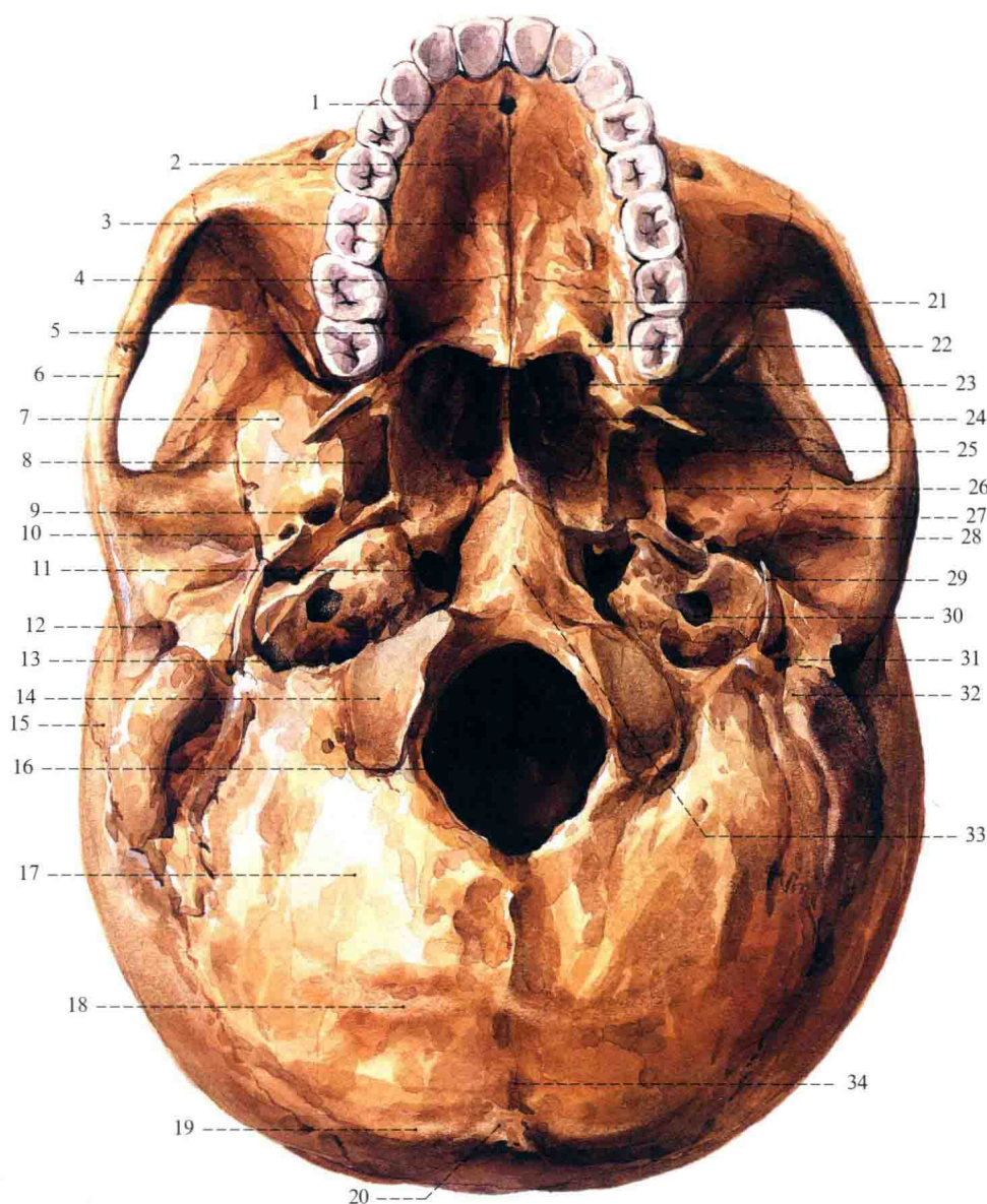
3. 颅底(下面观)
