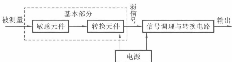
图 1-1 传感器的组成
