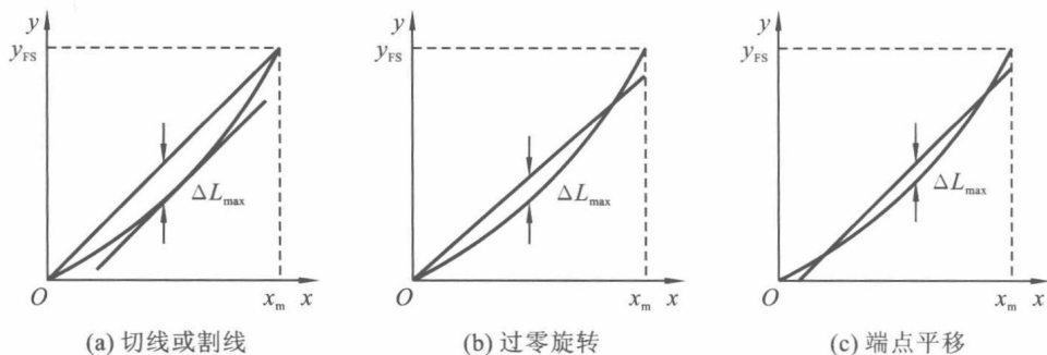
图 1-4 几种非线性拟合
