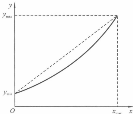
图 1-2 零输入-满量程输出拟合
