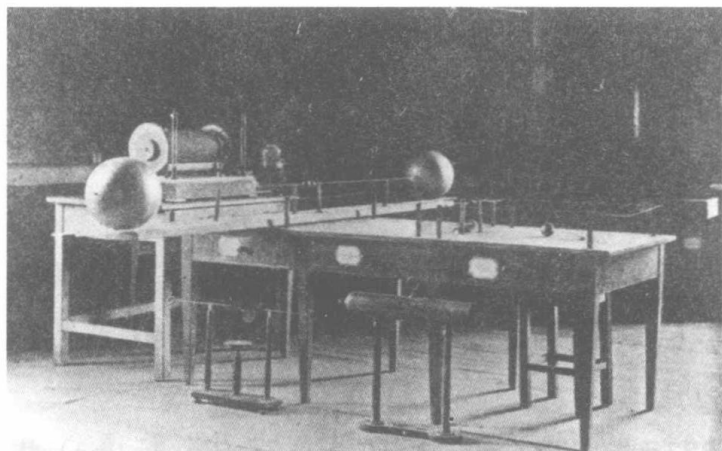
赫兹的装置 Schleiermacher 1901
