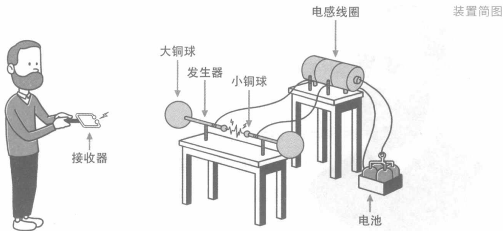
装置简图
