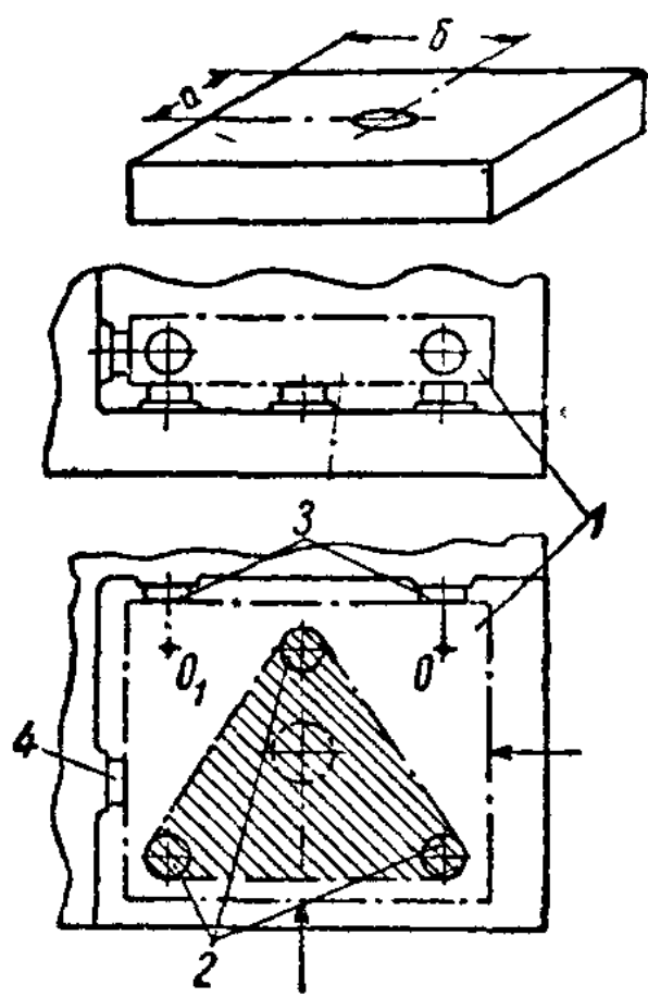
圖3 工件在六個支承上定位。
