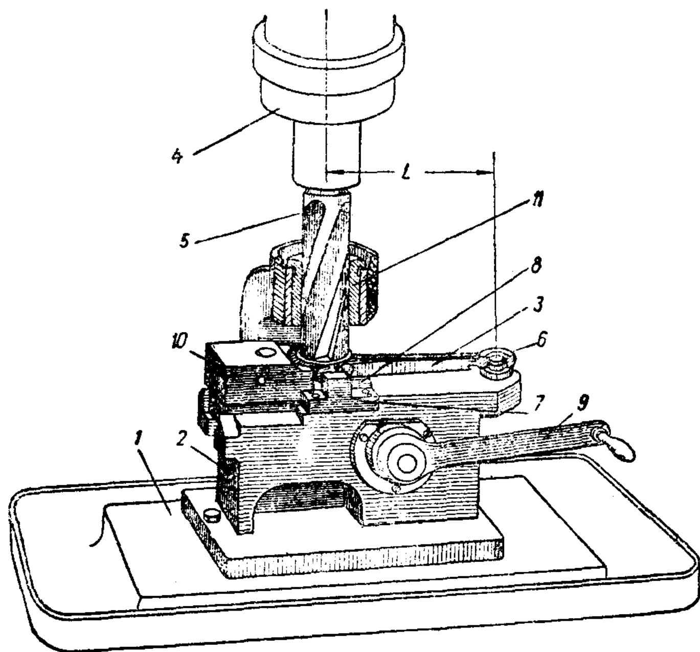
圖2 立式鑽床的工藝用具。
