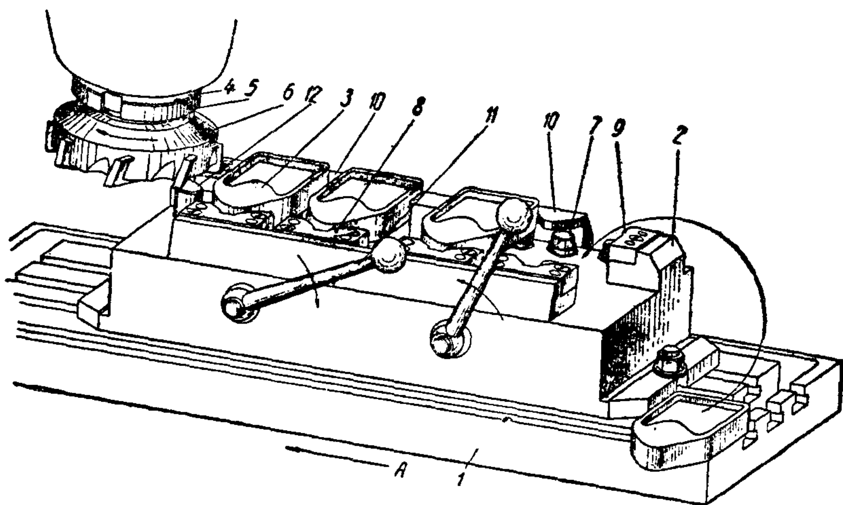
圖1 銑床的工藝用具。
