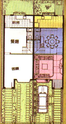
一樓平面圖
