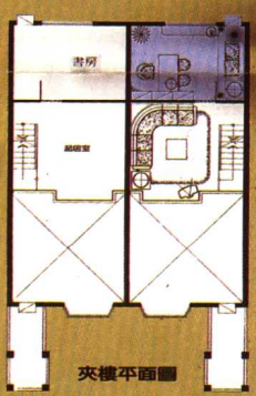
二樓平面圖
