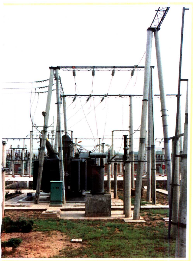
北庄 110 千伏变电站外景
