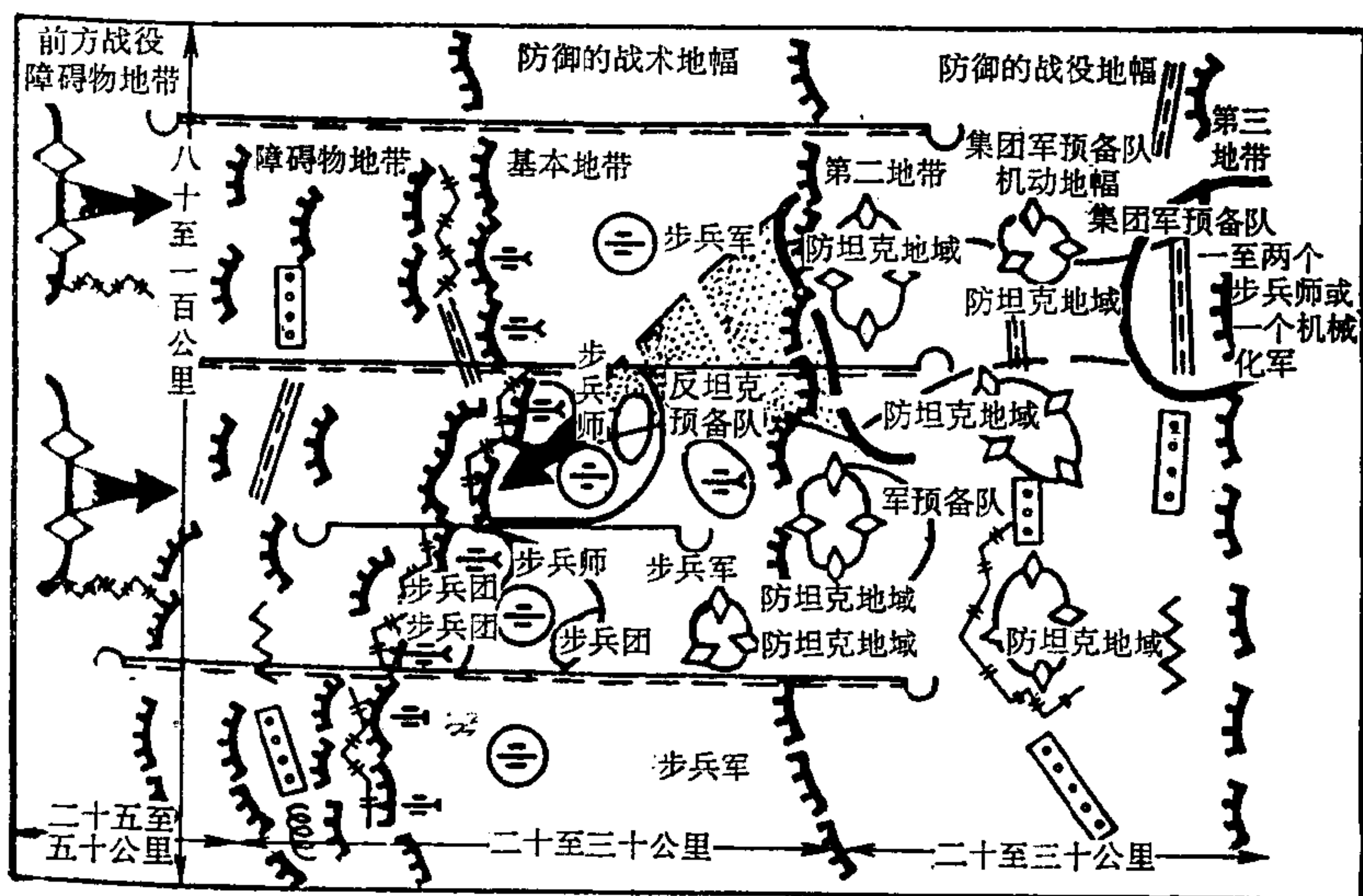
图16. 按战前观点集团军和步兵军的防御
