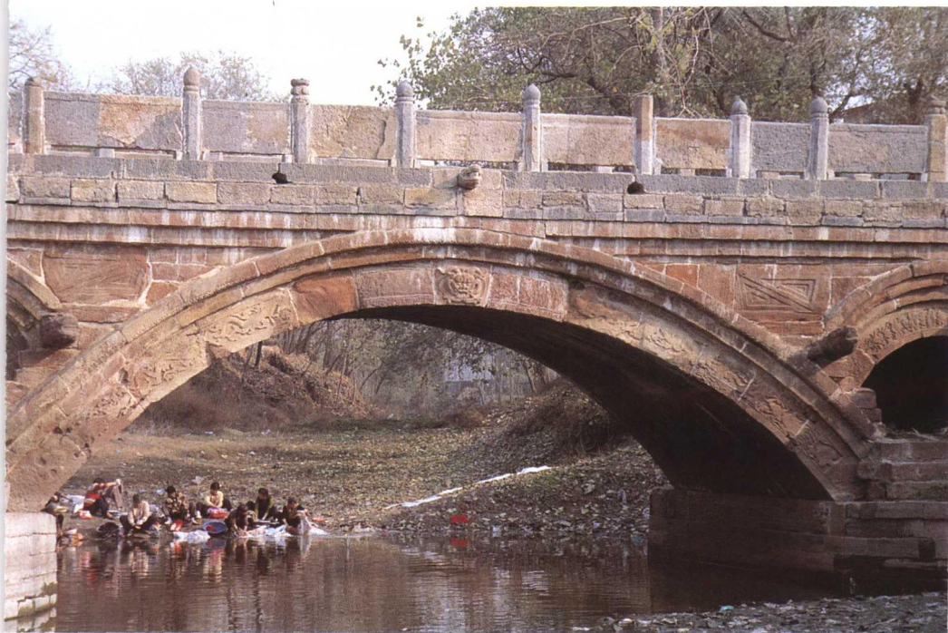
▲ 主拱券上游立面
