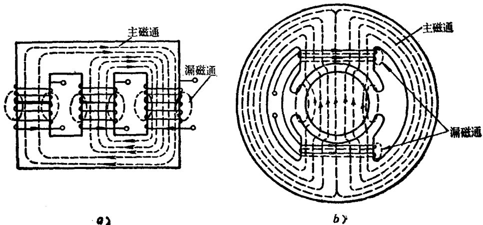
图 1-1 常见的两种磁路 a) 变压器的磁路 b) 二极直流电机的磁路
