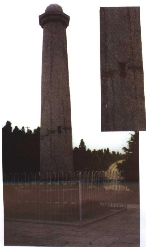
乾陵入口处华表腰身上的燕尾形细腰铁栓
