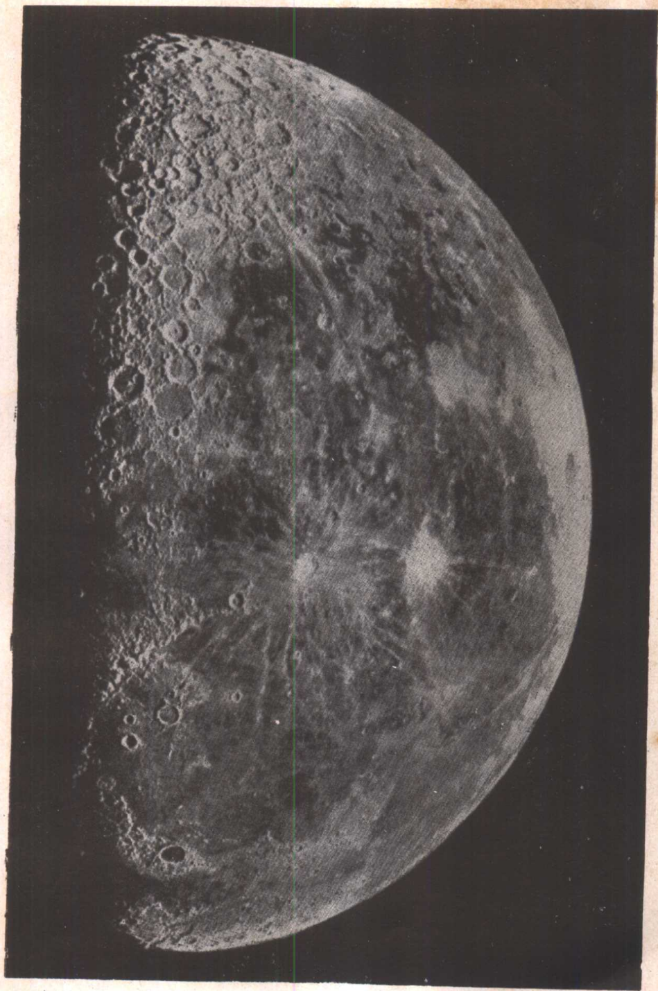
图 0.1 下弦时的月亮
