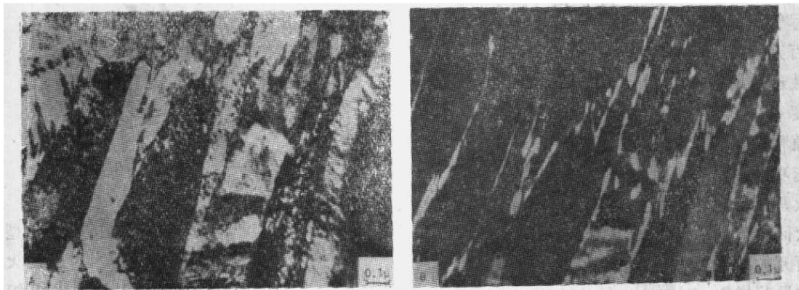
图 6 300-M 直接从 870°C 油淬的透射电子显微镜照片, 显示出残余奥氏体膜围绕在马氏体板条周界: (A) 明场成象; (B) 相反衬度的奥氏体反射暗场成象
