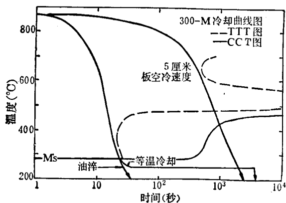
图 1 300-M 钢转变图所研究的几种冷却曲线示意图
