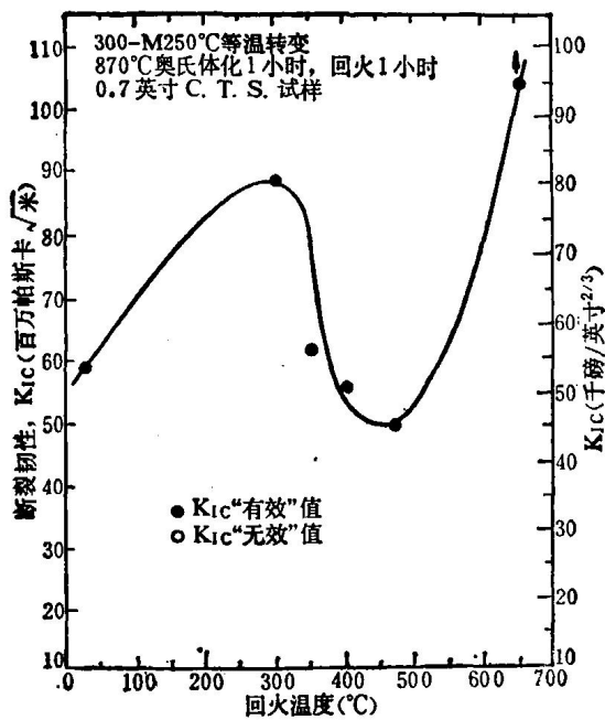
图9 回火温度对250°C等温1小时处理的300-M钢室温平面应变断裂韧性的影响
