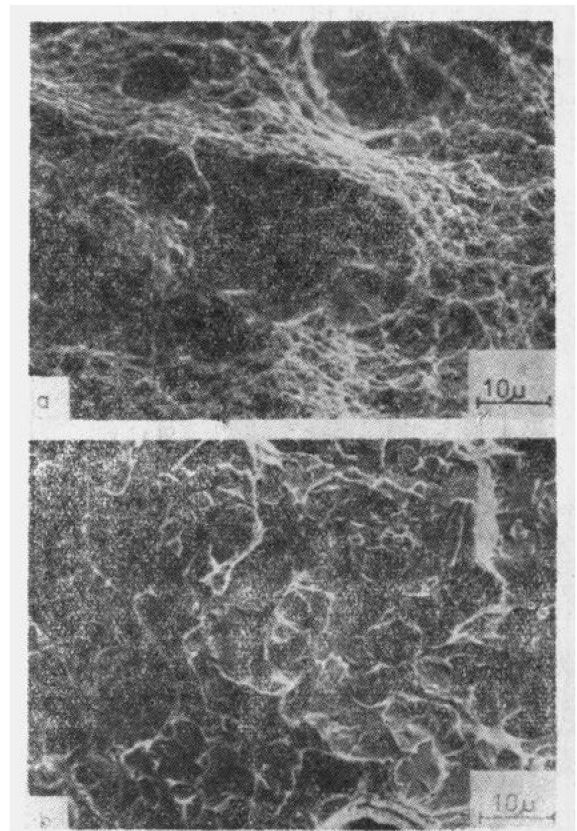
图 16 空冷 4340 钢破坏机构, (a) 200°C 回火, 显示延性断裂, (b) 275°C 回火, 显示穿晶解理
