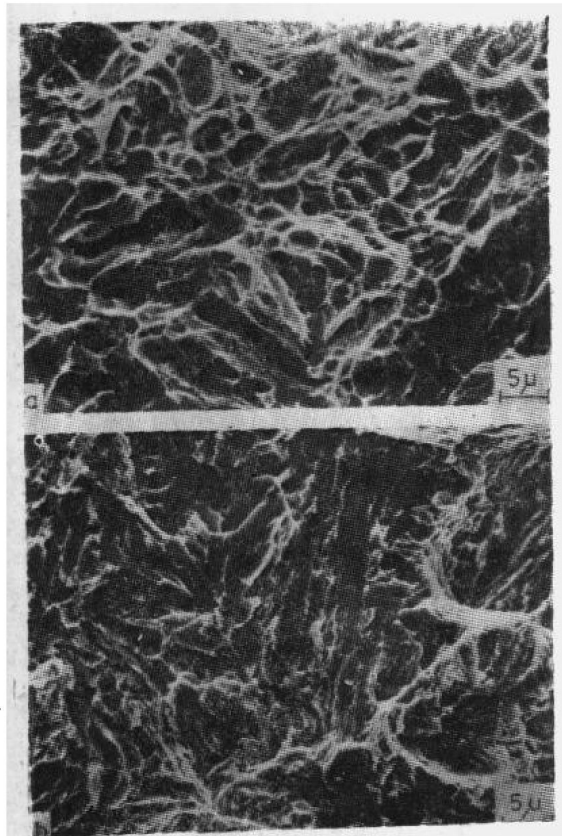
图10 经等温处理的300-M破坏机构, (a) 300°C回火显示延性断裂, (b) 470°C回火显示板条间解理
