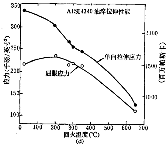
图2 回火温度对所研究几种热处理室温下单向拉伸性能的影响。
