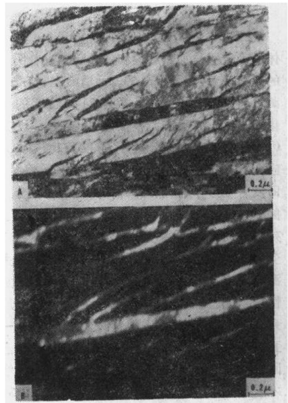
图11 300-M空冷,300°C回火的透射电子显微镜照片,显示出贝氏体-马氏体基体上有残余奥氏体膜:(A)明场成象;(B)相反衬度奥氏体反射暗场成象
