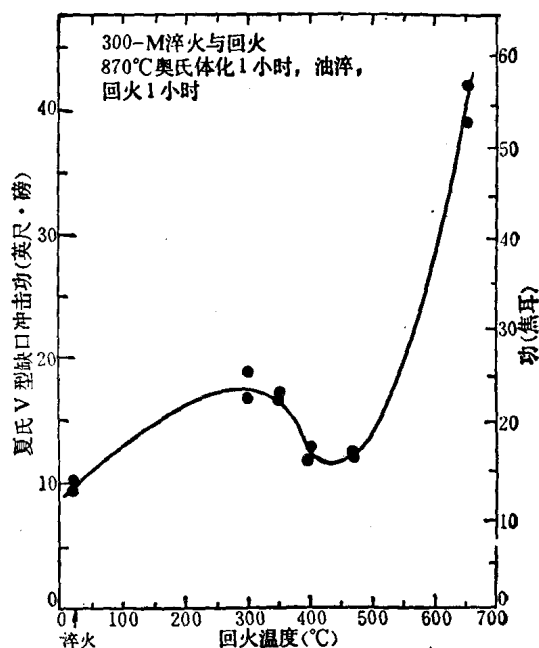
图4 回火温度对300-M钢油淬后室温夏氏V型缺口冲击功的影响
