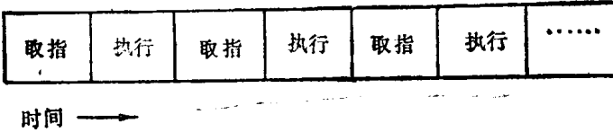
图 2-2 8080/8085程序执行顺序
