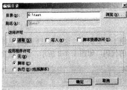
图 1-2-7 “编辑”目录
