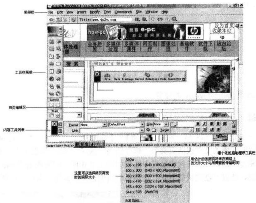
图 1-3-1 UltraDev 主界面
